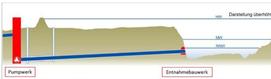
Schnitt: Anordnung von Pumpstation und Entnahmebauwerk
