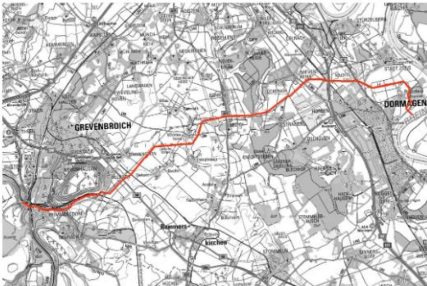
Geplanter Verlauf der Rheinwassertransportleitung
