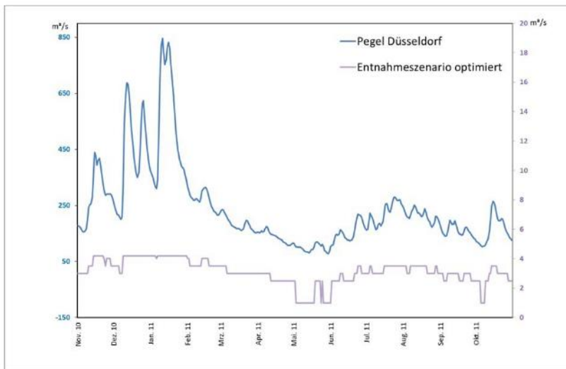
Abbildung: Wasserstandsabhängige Entnahme
